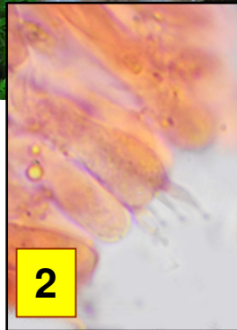
1 : Spores 6-9,5 x 5-5 \mu m, cylindro-elliptiques 2 : Cystides tétrasporiques.
