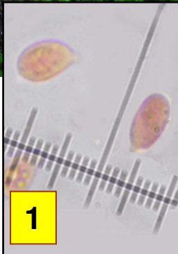
1 : Spores 6-9,5 x 5-5 \mu m, cylindro-elliptiques 2 : Cystides tétrasporiques.
