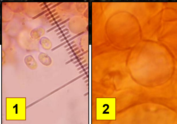
1 : Spores 5,5-5 x 2-2,5 \mu\text{m} , elliptiques ou ovoïdes. 2 : Revêtement piléique en épithélium.
