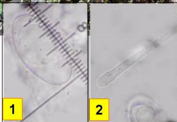
1 : Spores largement ellipsoïdes, lisses, hyalines, 18-22 \times (10) 13-15 \mu\text{m} . 2 : Paraphyses élancées, septées, ramifiées vers la base, légèrement clavées à l'apex.
